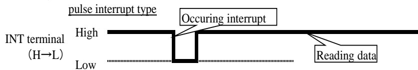
Fig.11 Interrupt output (pulse interrupt type )
