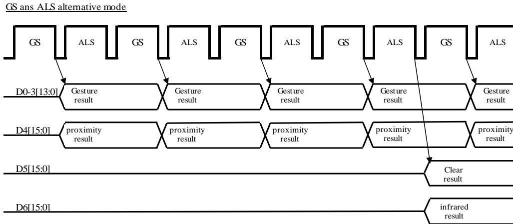
Fig.8 Output results for GS/PS and ALS alternating mode
